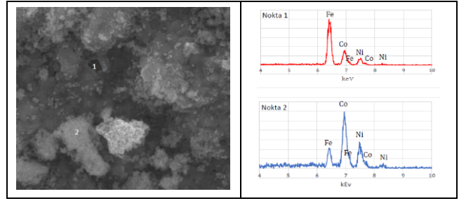
Ek A1: İki farklı noktadan alınan SEM-EDS analiz spektraları (4-10 keV aralığında). Koyu renkli bölgeler demir zengin (kobalt ve nikel fakir) açık renkli bölgeler ise demir fakir (kobalt ve nikel zengin).
