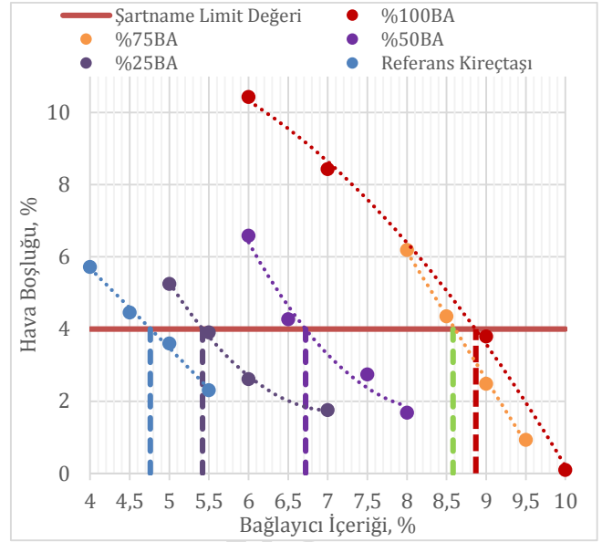
Şekil 1: Hava boşluğu-bitüm grafiği
