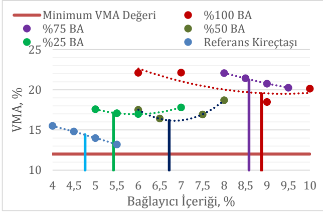
Şekil 2: VMA-bitüm grafiği
