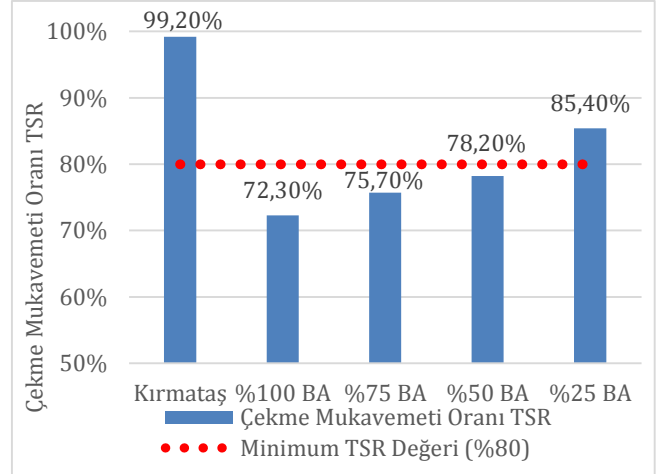
Şekil 5: Çekme mukavemeti oranı değerleri
