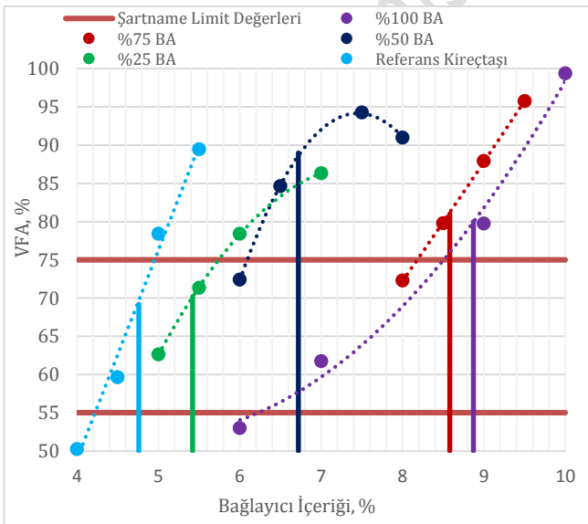
Şekil 3: VFA-bitüm grafiği
