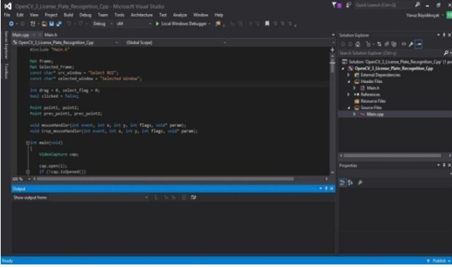
Şekil 1: Kullanıcı arayüzü
