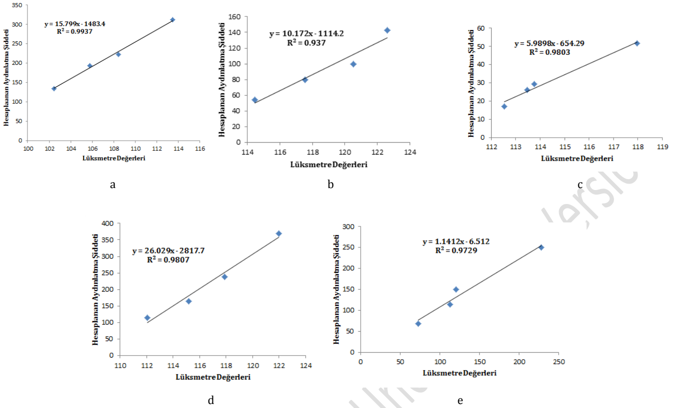
Şekil 8: a,b. LED aydınlatma, c,d. Akkor aydınlatma e.Fluoresan aydınlatma için ölçüm sonuçları ile hesaplama sonuçları arasındaki ilişki örnekleri
