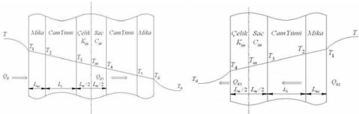
Şekil 2. İç ve Dış Duvar kesitleri
