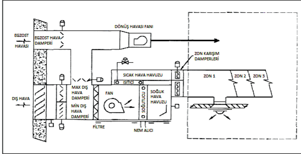
Şekil 1. Çok bölgesli iklimlendirme sistemi (Başer, 2006)
